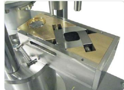
4 MORDAZAS APRIETA-CORCHO
